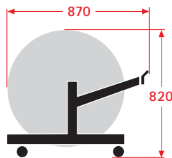
Untertisch-Schneidgerät, fahr- und arretierbar Under-worksurface cutter, mobile and lockable Appareil de coupe sous table, mobile avec dispositif de blocage Best.-Nr. / Ref. / Réf. 255...
